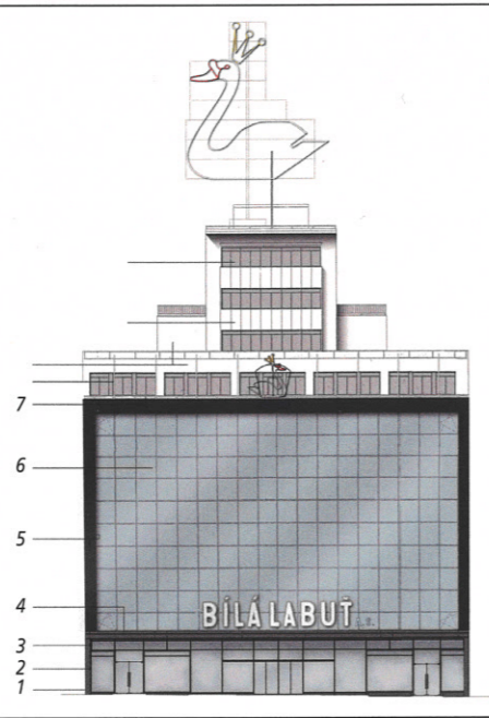
Detail řešení uliční fasády – keramický obklad zateplené fasády v původním rastru 65 x 65 mm
