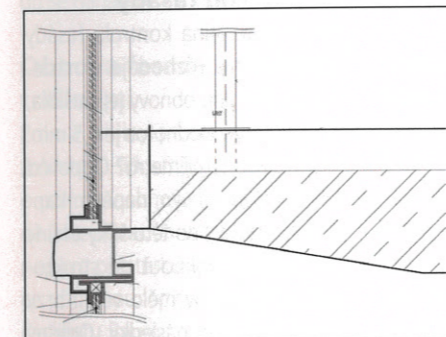
Uchytení stropní desky – původní řešení
