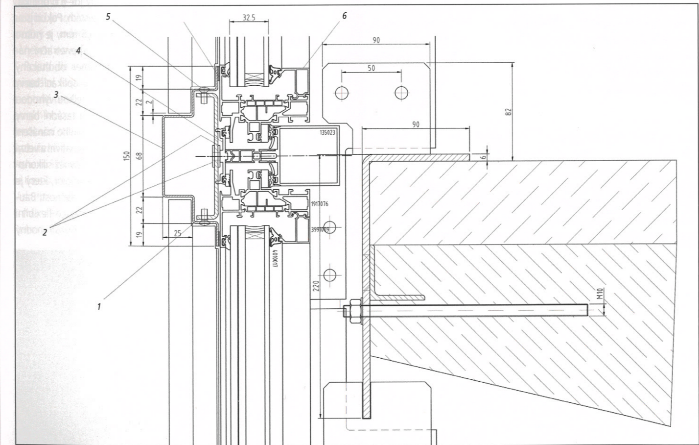
Uchytení stropní desky:
